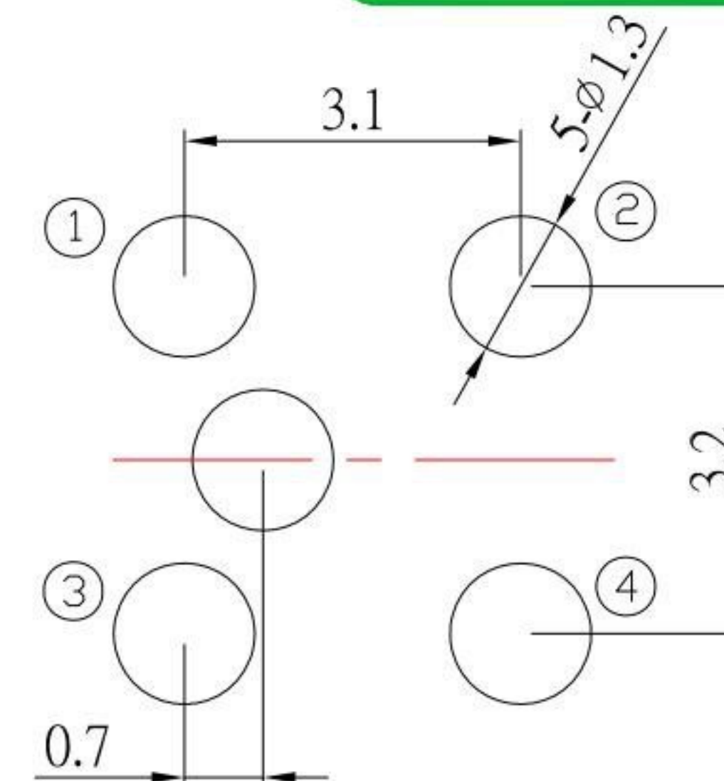
P.C.B LAYOUT
