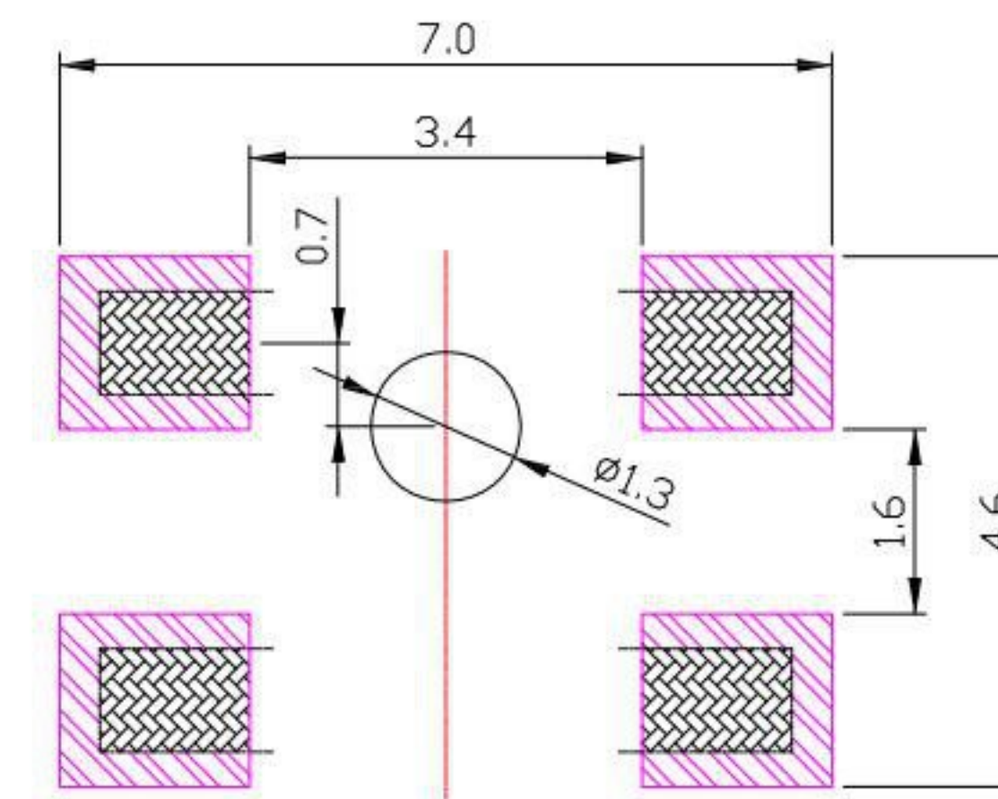
P.C.B LAYOUT
