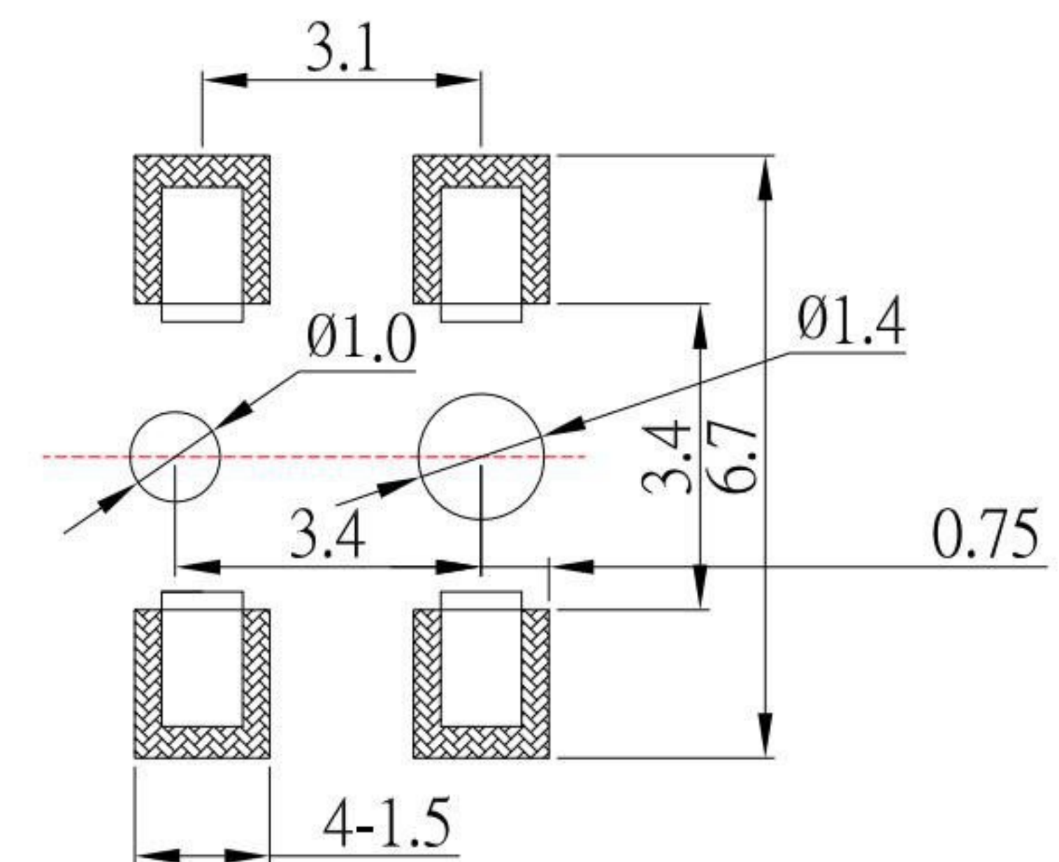
P.C.B LAYOUT
