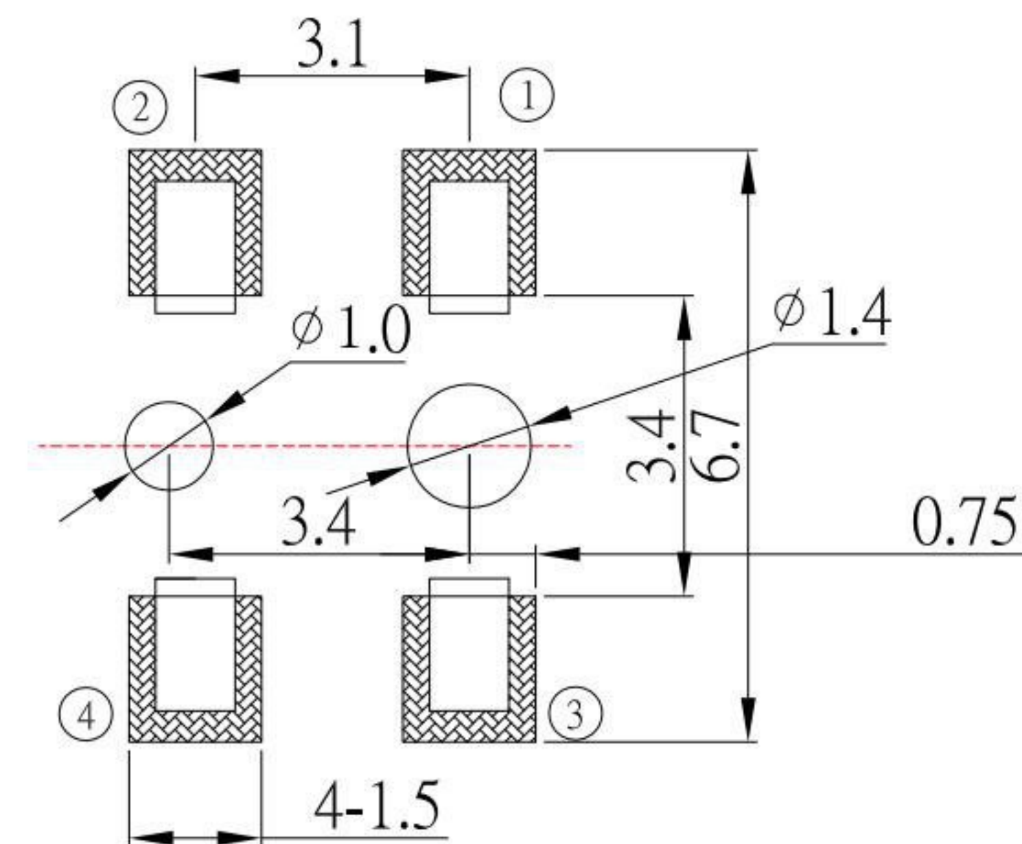
P.C.B LAYOUT
