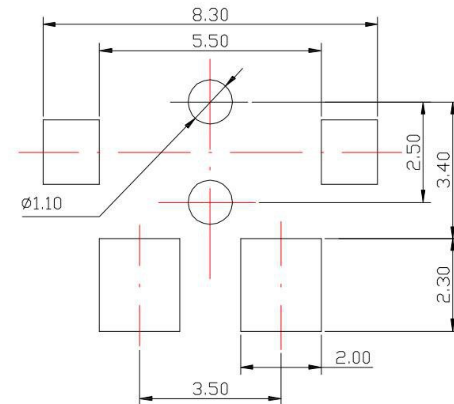
P.C.B LAYOUT
