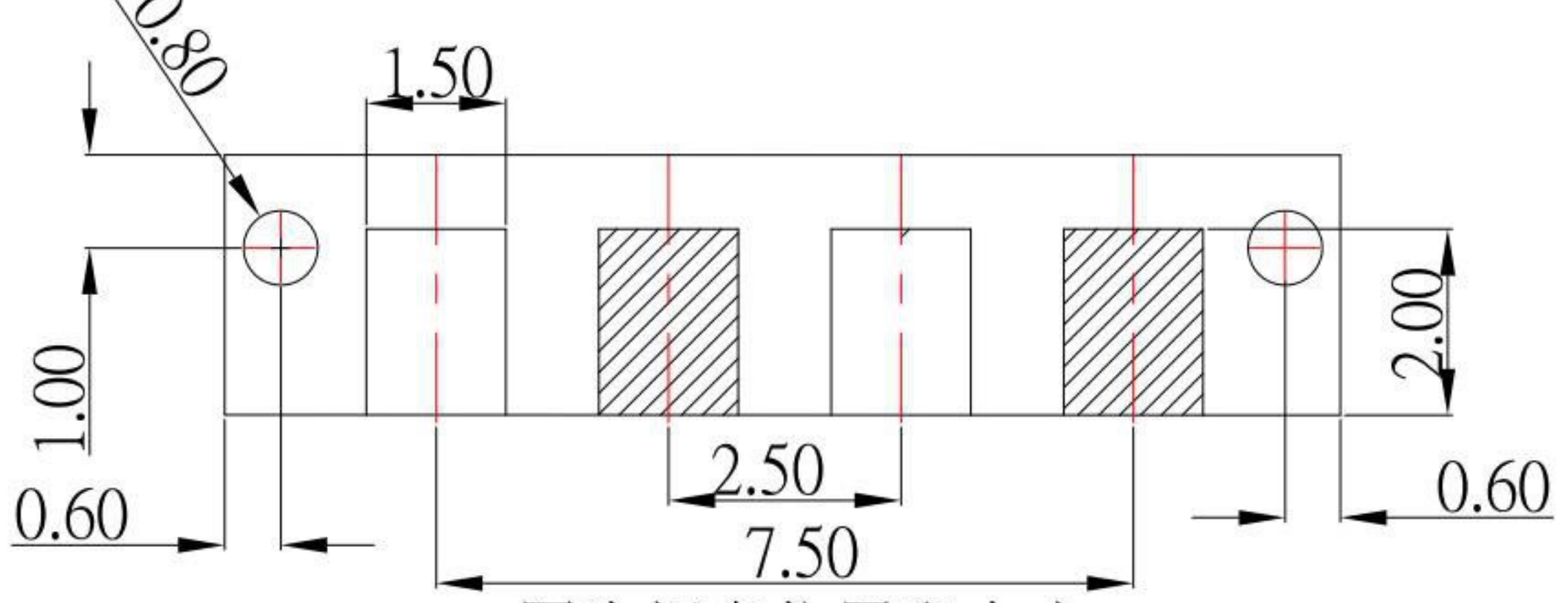
图为焊盘位置和大小
