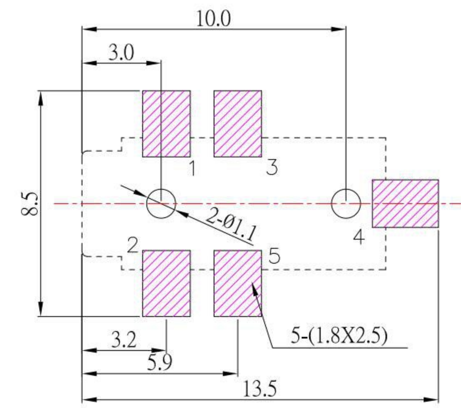
P.C.B LAYOUT
