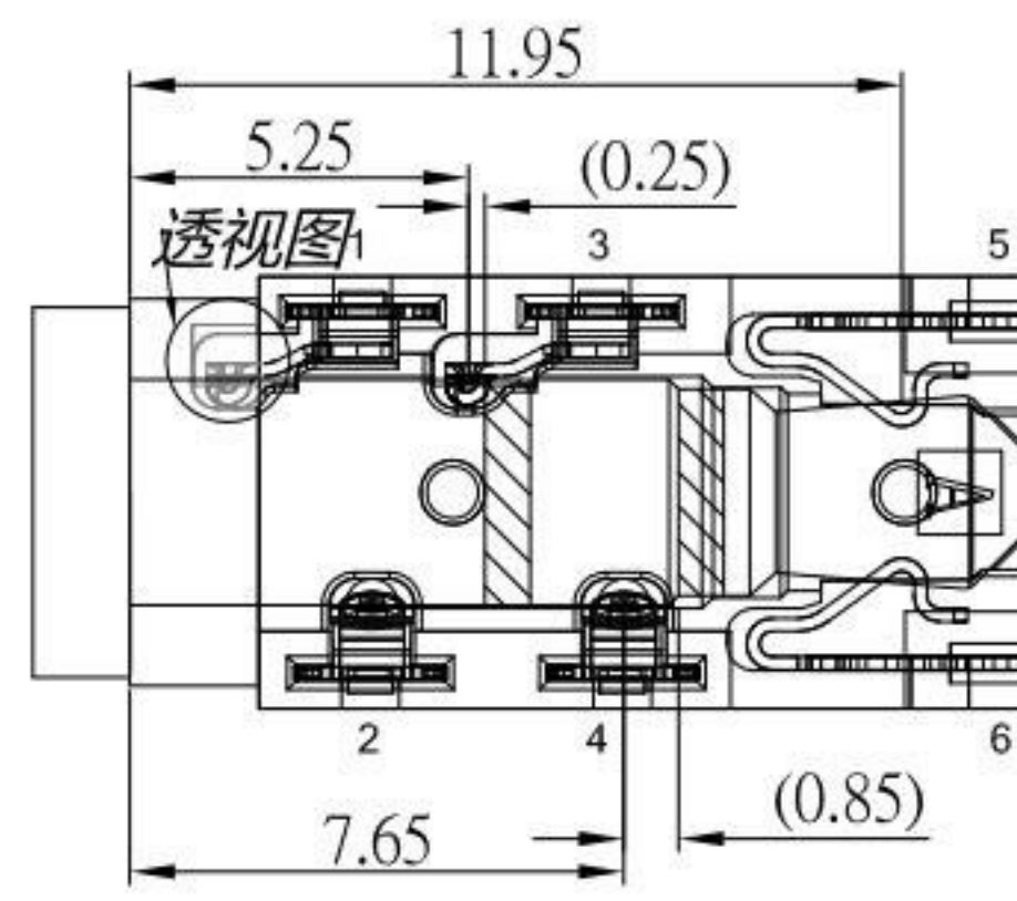
3 级插头接触点位置尺寸
