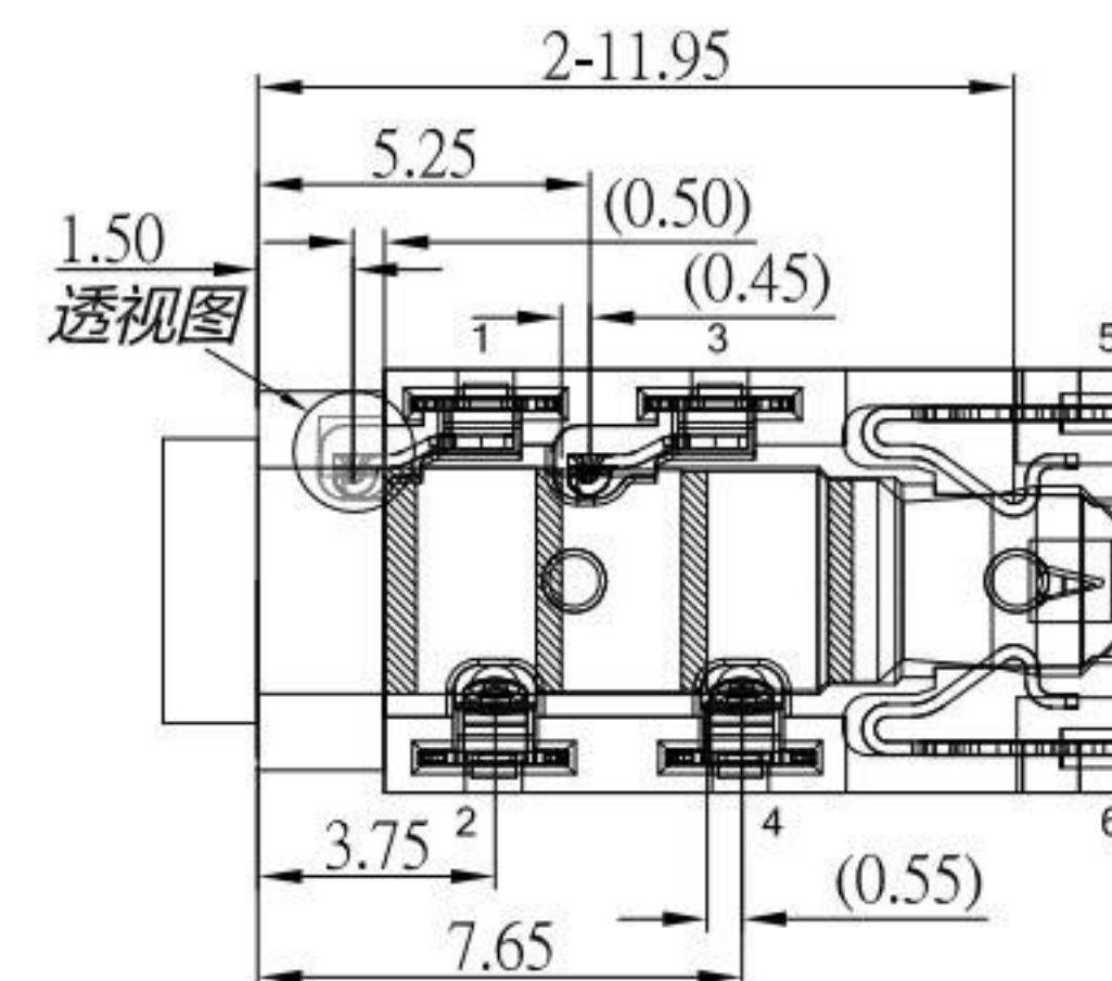
5 级插头接触点位置尺寸
