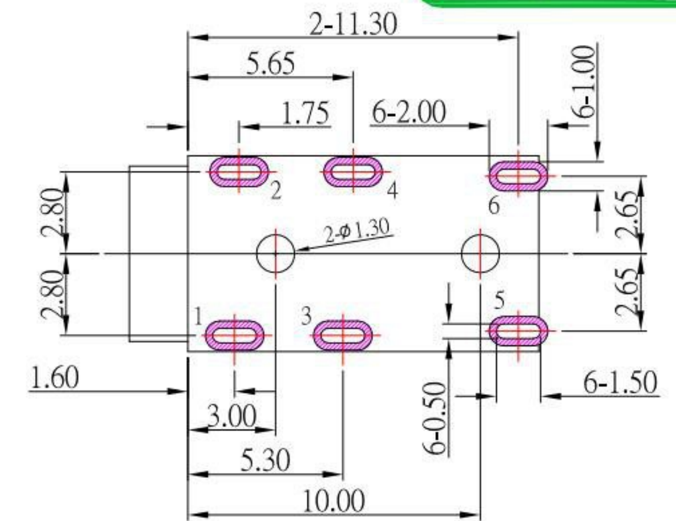
P.C.B LAYOUT
