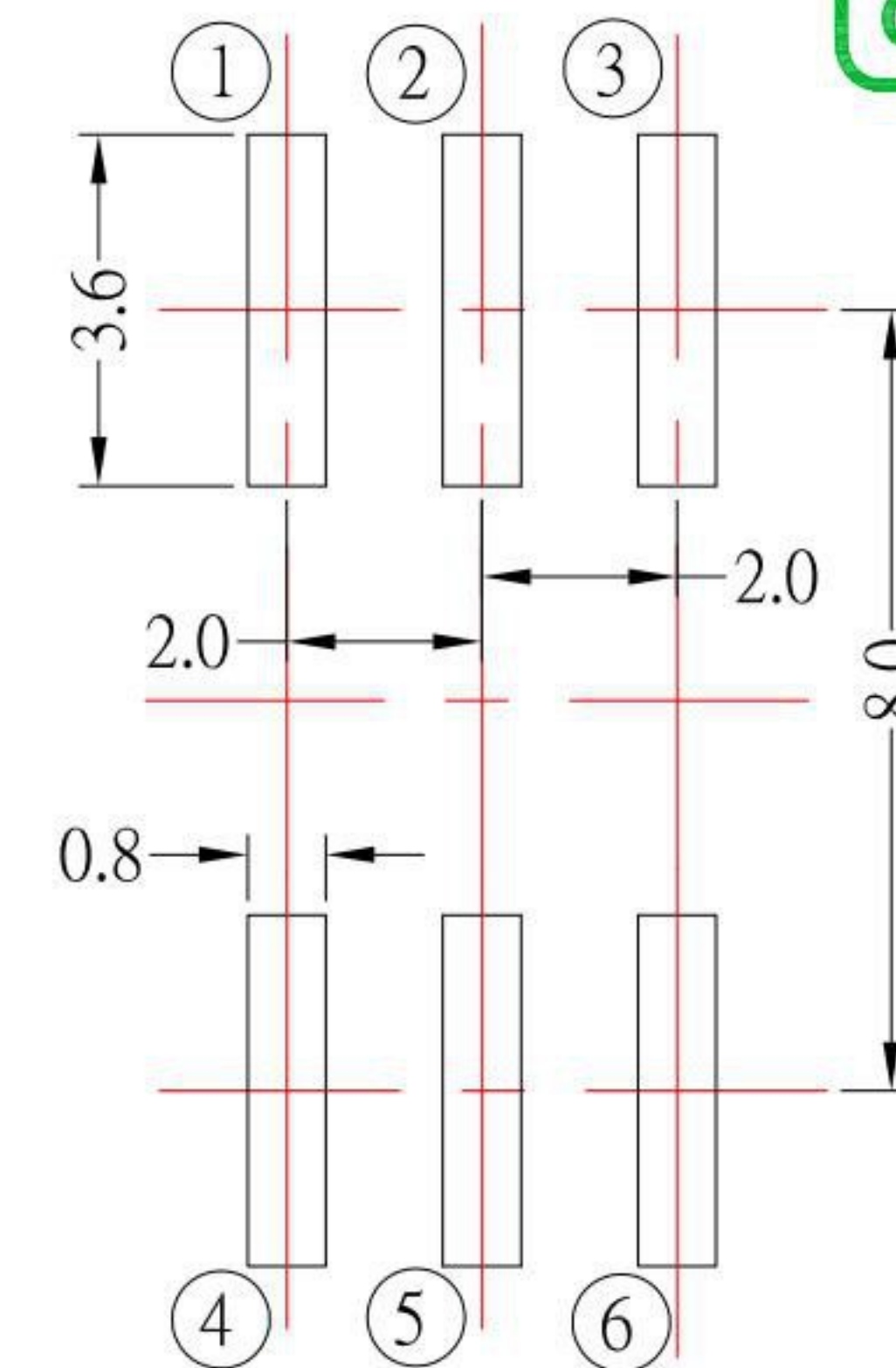
P.C.B LAYOUT
