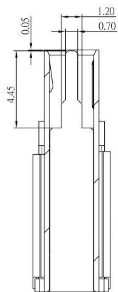
剖視圖
