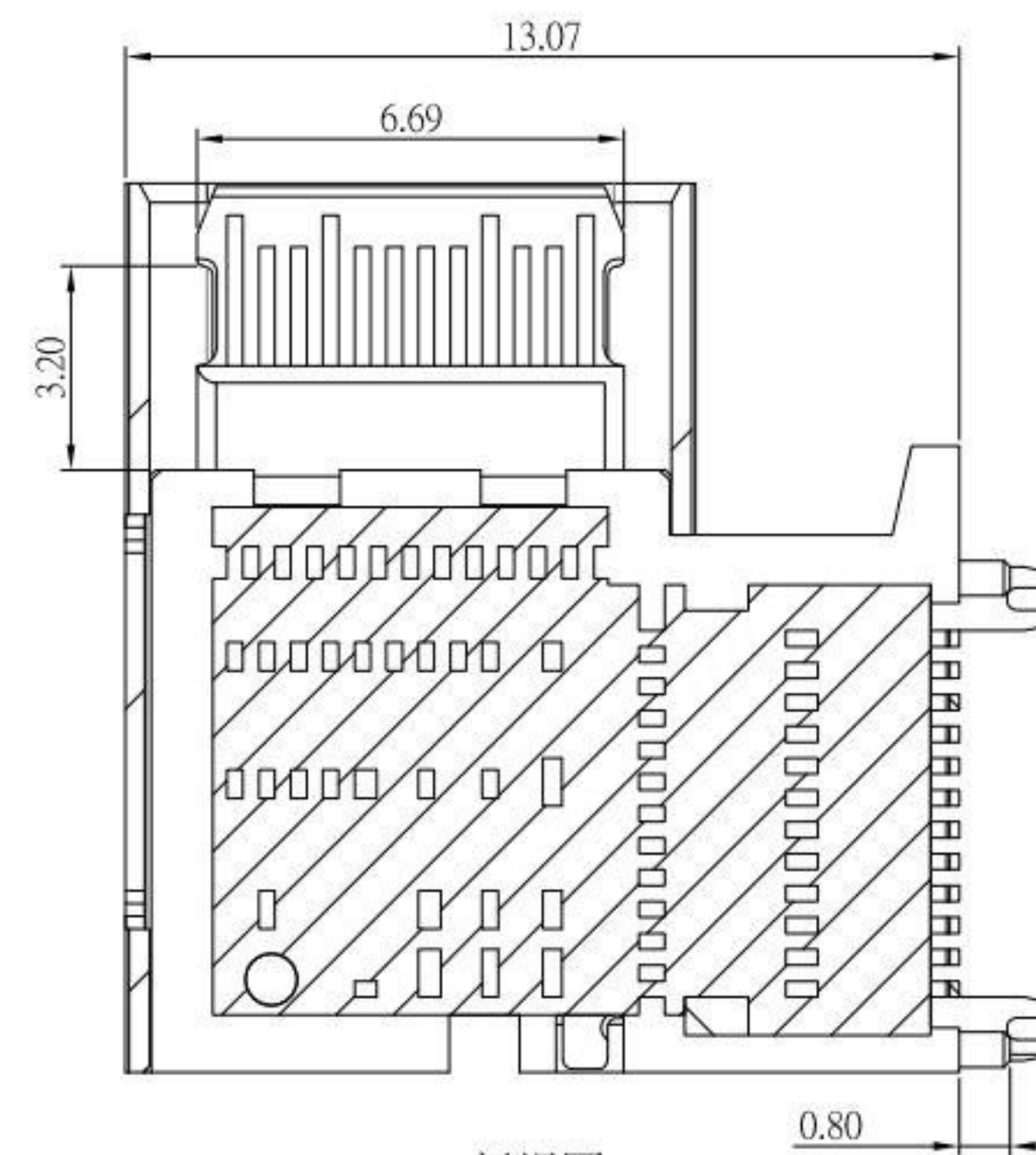
剖視圖
