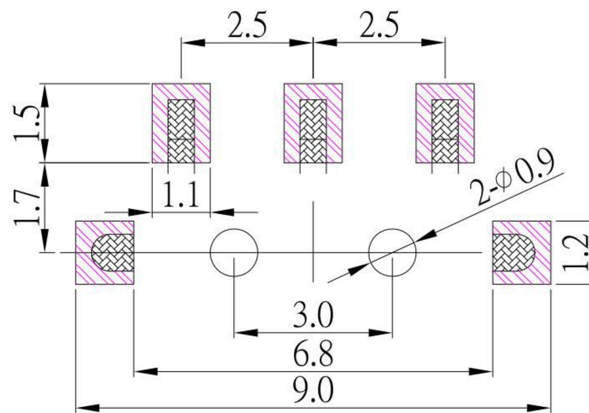
P.C.B LAND PATTERN
