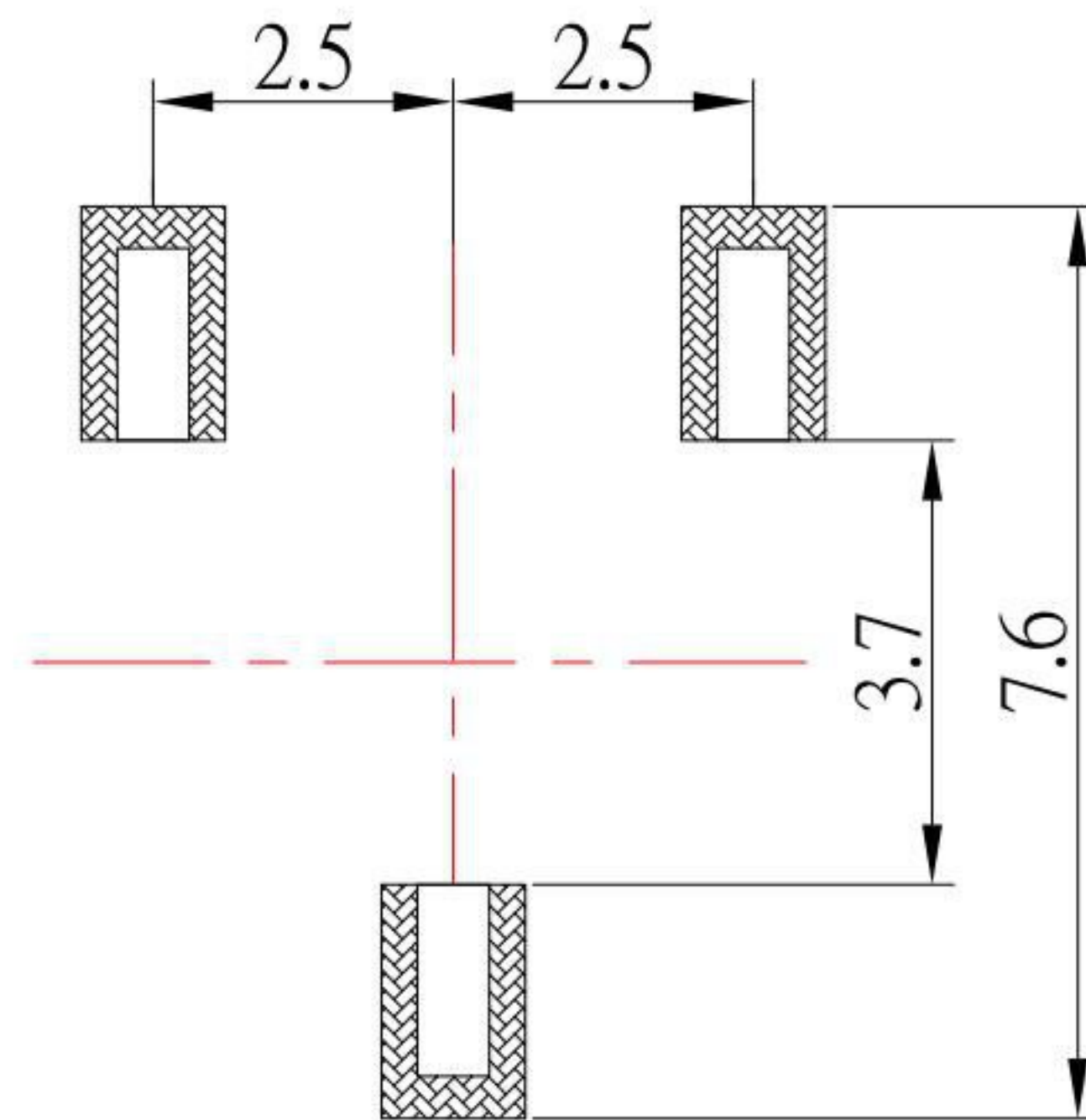
P.C.B LAND PATTERN
