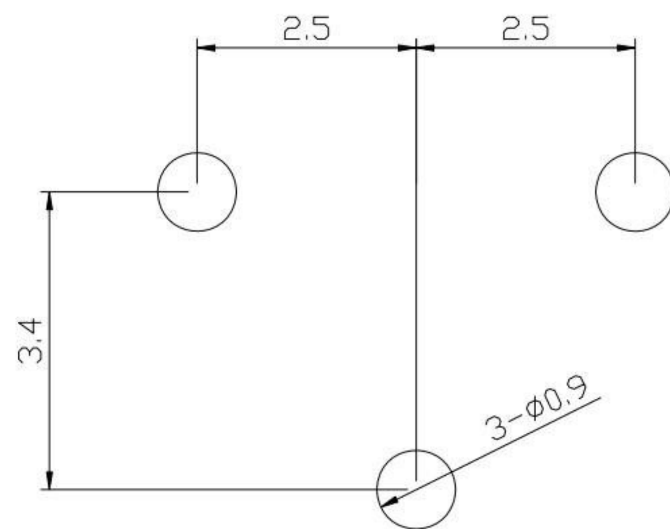
P.C.B LAND PATTERN
