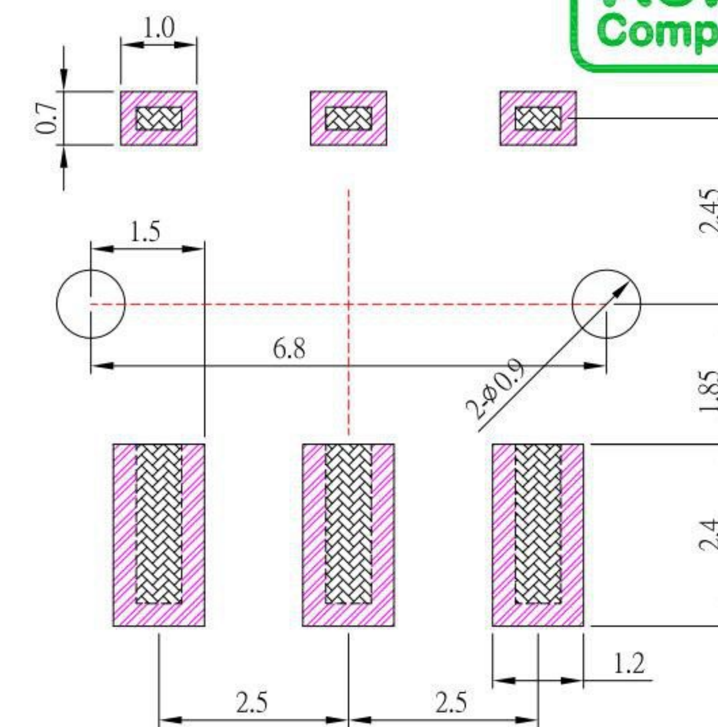
P.C.B LAND PATTERN
