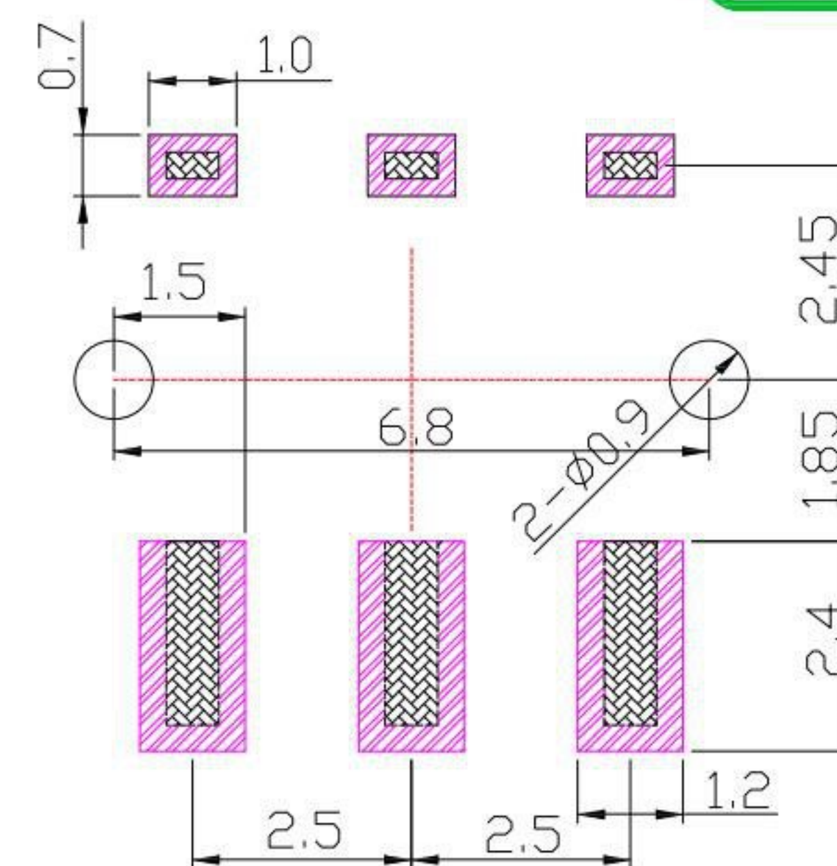
P.C.B LAND PATTERN
