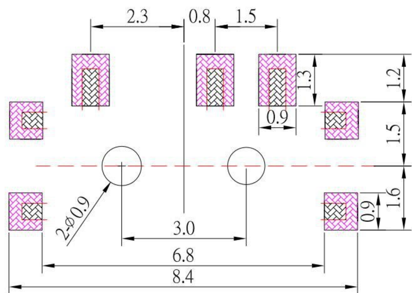
P.C.B LAND PATTERN
