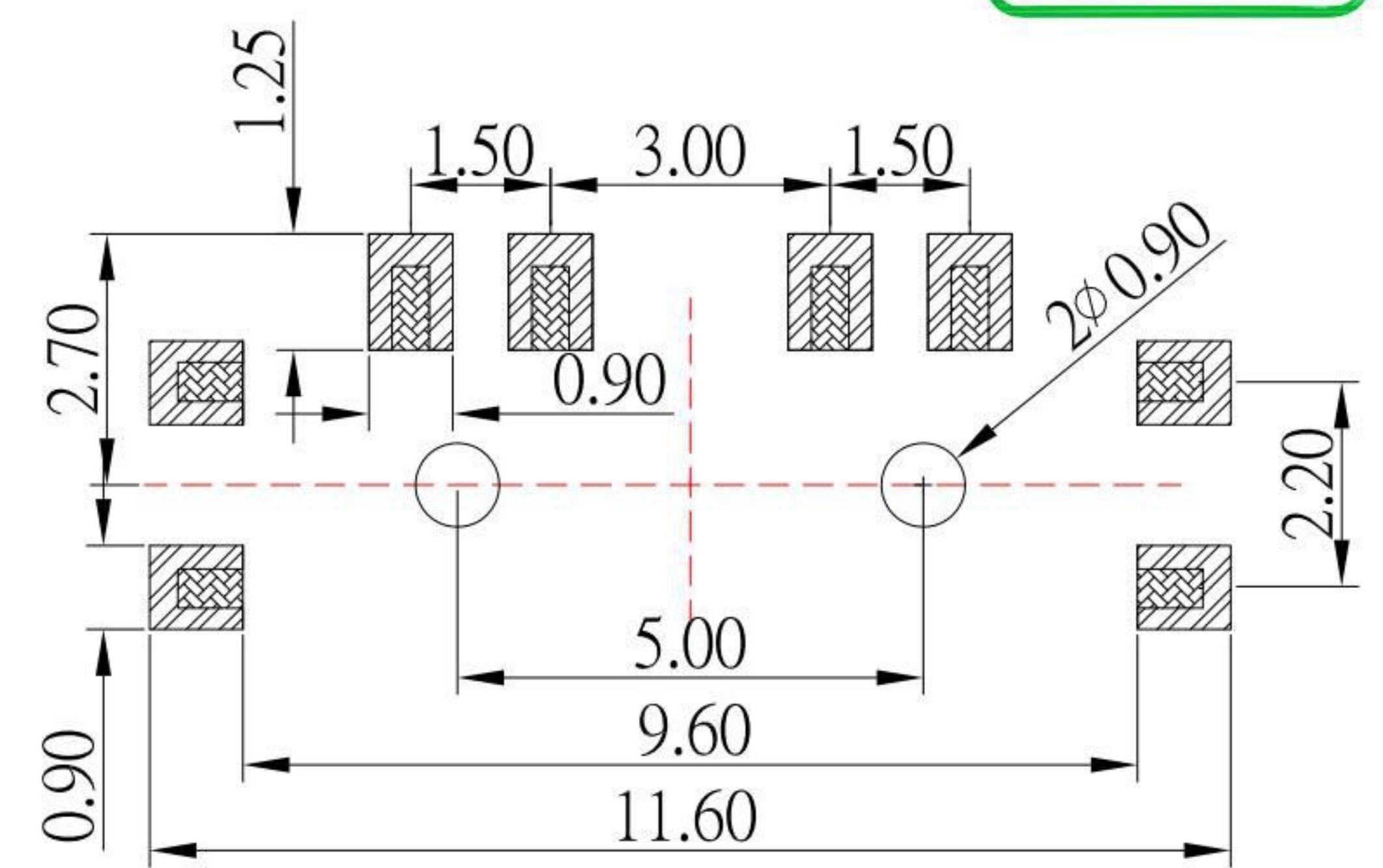
P.C.B LAND PATTERN
