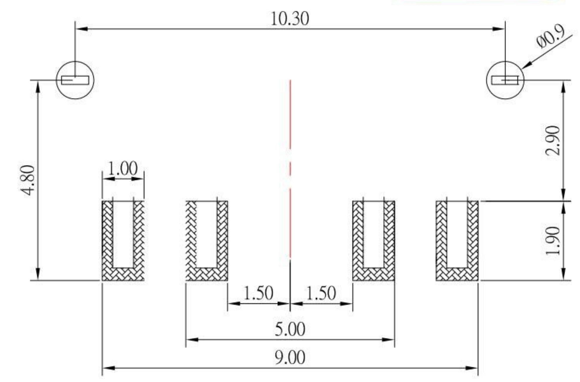
P.C.B LAND PATTERN
