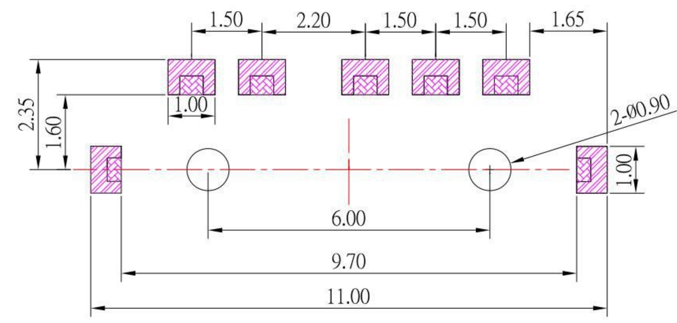
P.C.B LAND PATTERN
