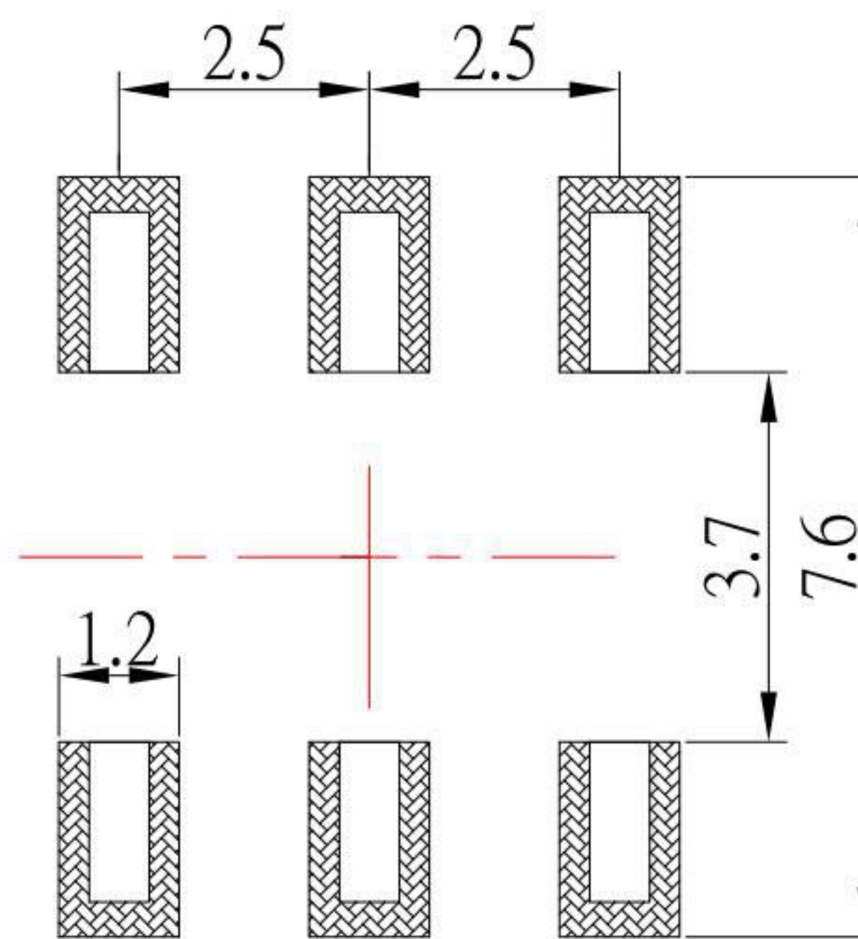
P.C.B LAND PATTERN
