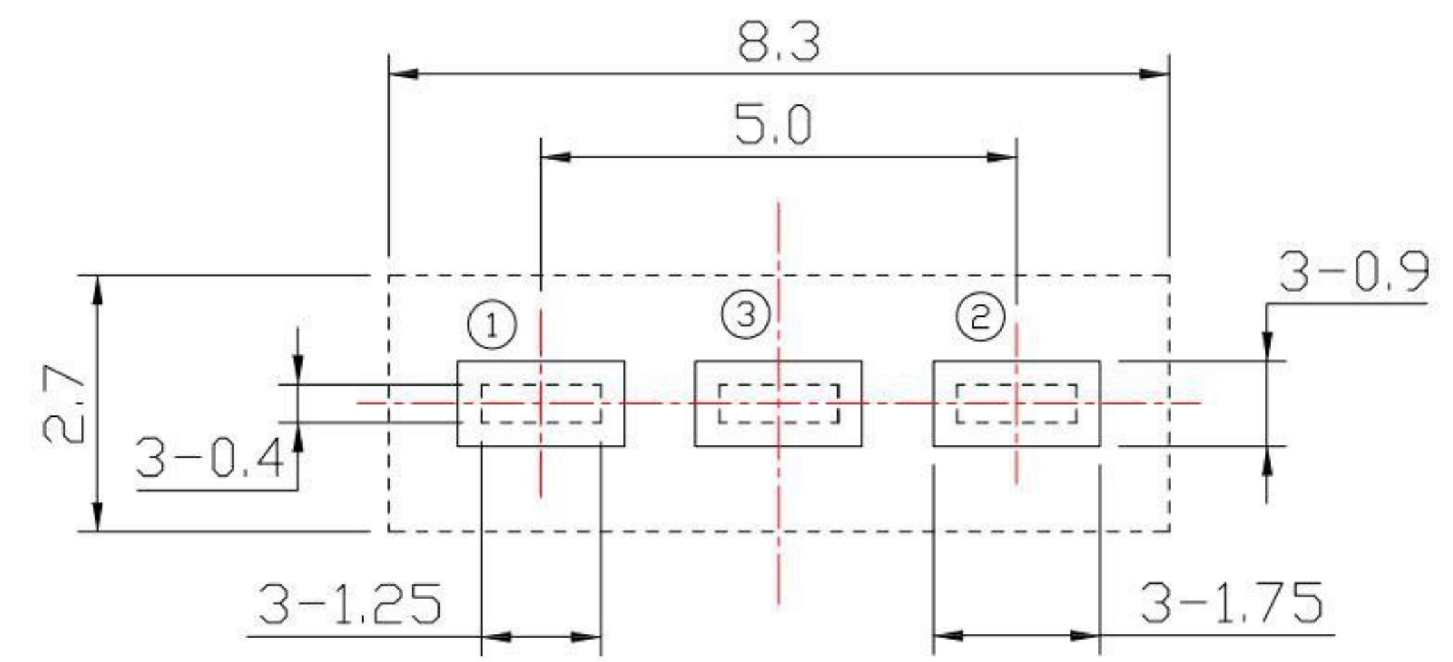
P.C.B LAYOUT
