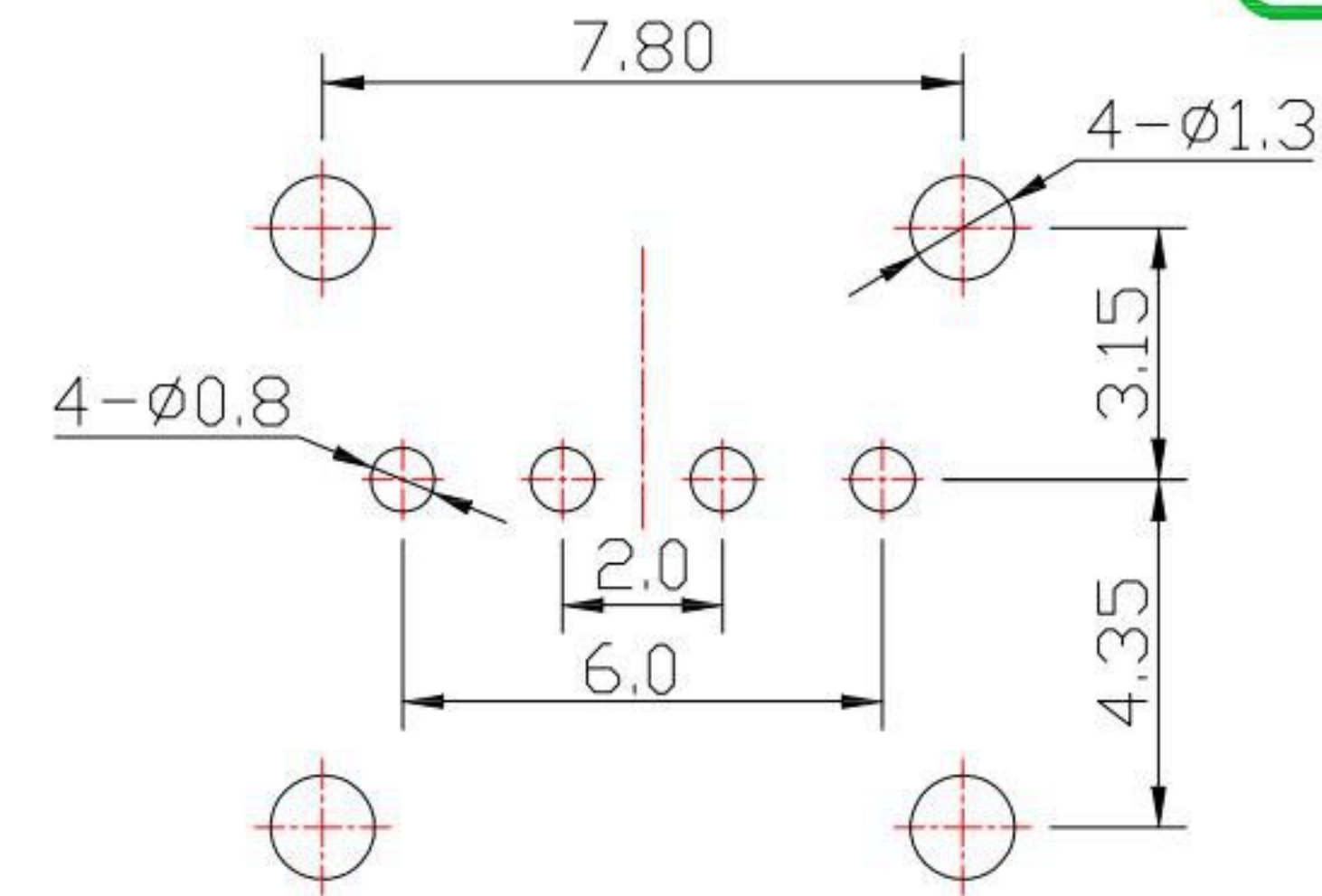
P.C.B LAND PATTERN
