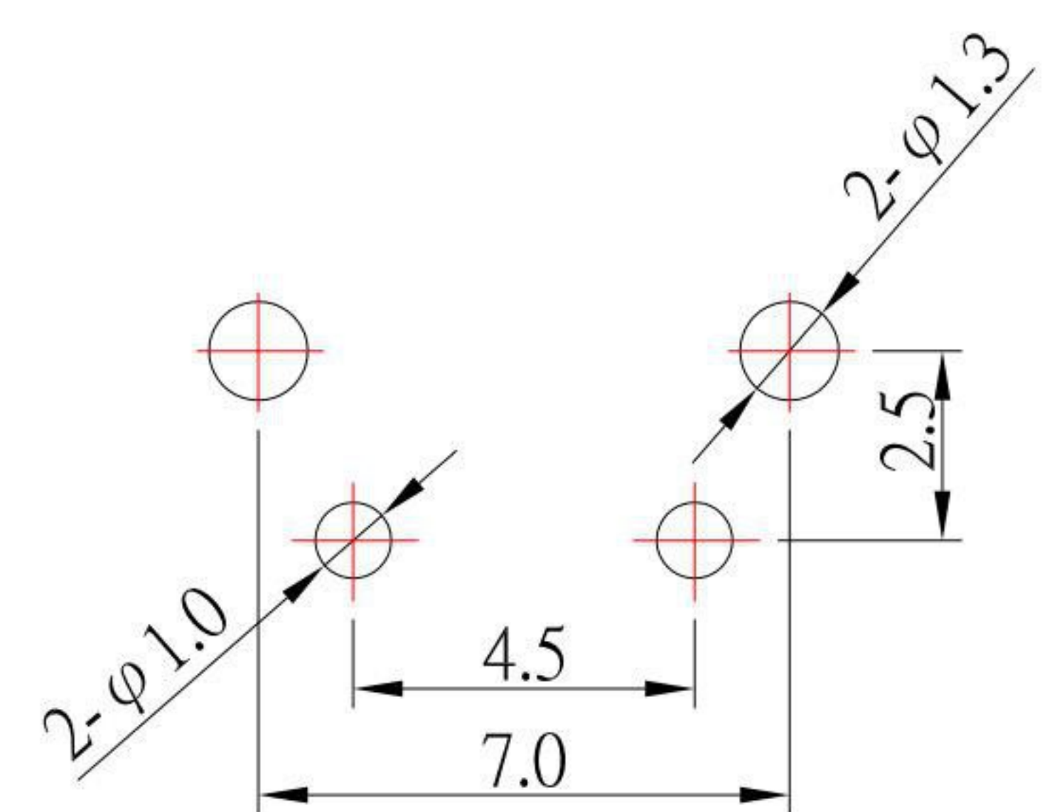
P.C.B LAYOUT
