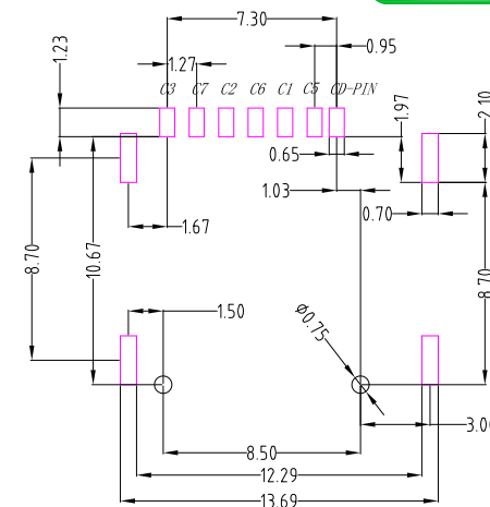
P.C.B LAYOUT
