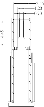
截面 2-2
